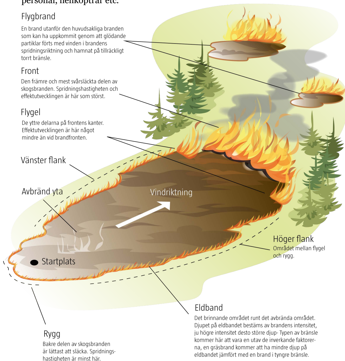
Figur 1. Skogsbrandens delar
