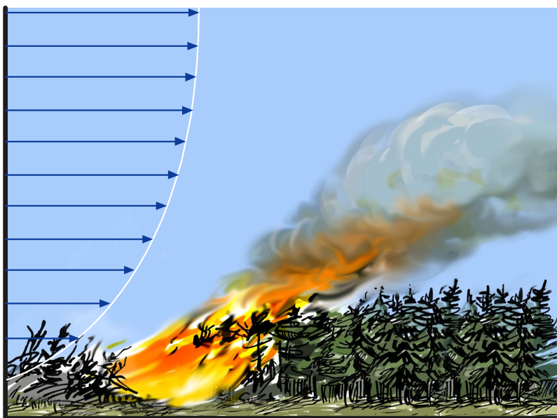
Figur 2. Vindburen toppbrand kan uppkomma när vindstyrkan ökar och brandgaser från brinnande träd antänder angränsande trädtoppar.
