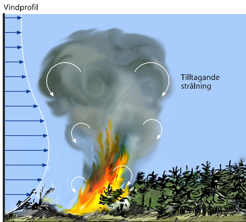
Figur 3. För att ett brandplymsdominerat brandförlopp ska uppstå krävs en stor mängd bränsle och mycket låg bränslefukthalt.
