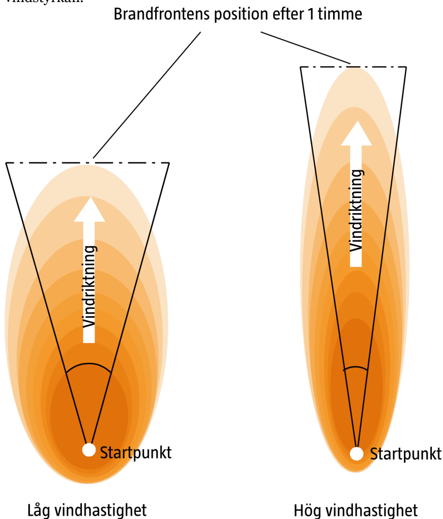
Figur 4. Skogsbrandens utbredning vid olika vindhastigheter.
