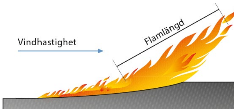
Figur 13. Flamlängd.
